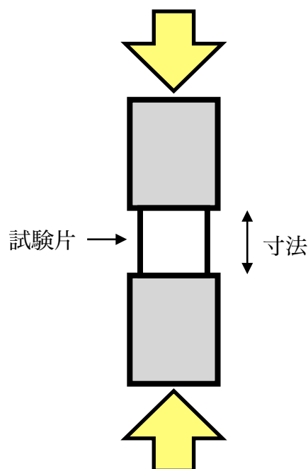
図 1.1 圧縮試験。加えた力と変位（寸法の変化）を同時に測定する。力の強さを断面積で割った値（応力または応力度）と変位の関係を記録する。
